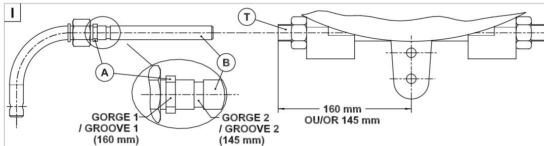
MONTAGE "DESSUS" LE LEVIER MOTEUR INSTALLATION "ABOVE" MOTOR LEVER
