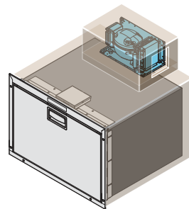
Fig. 2 Esempi di installazione con posizioni differenti dell'unità refrigerante Installation examples with different cooling unit positions
