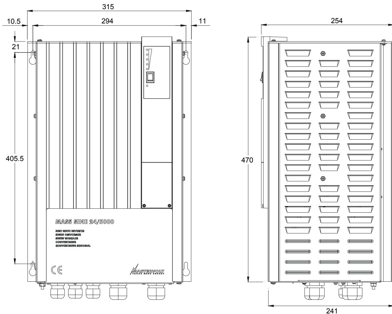
Figura 5: Dimensioni Mass Sine 24/5000- 230V
